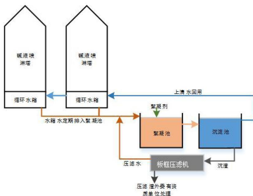
图 6.2-6 二级碱液喷淋处理工艺示意图
