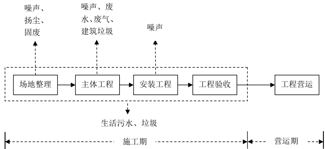
图 3.7-1 施工期工艺流程及产污节点图
