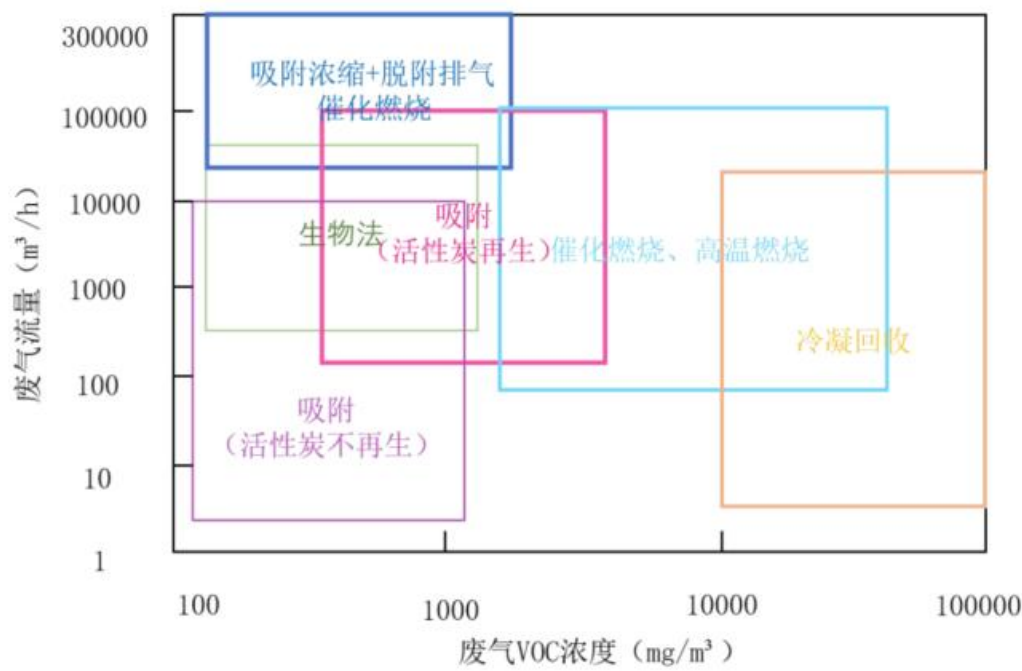
图 6.2-4 VOCs 治理技术适用范围（浓度、风量）
