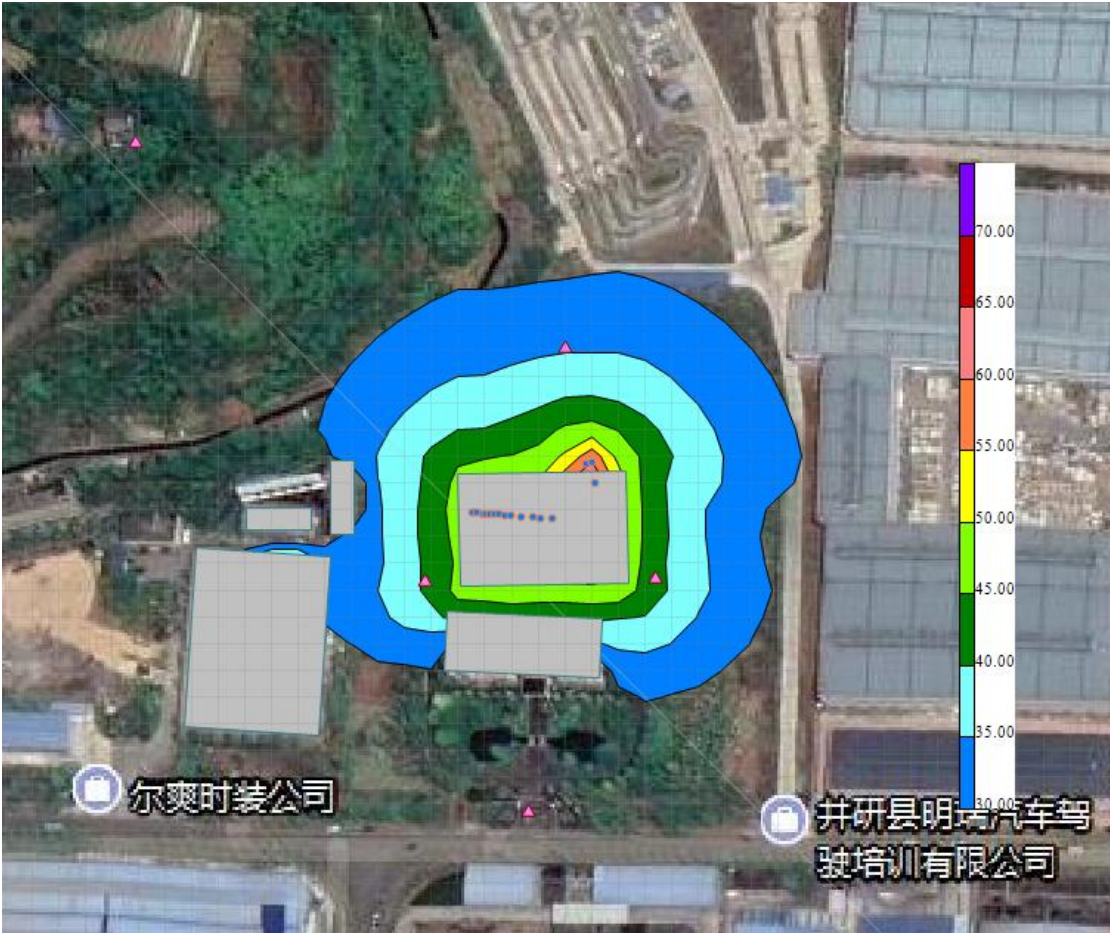
图 5.2-7 项目昼夜间噪声预测等声级线图（项目 24h 运行，昼夜间一致）
