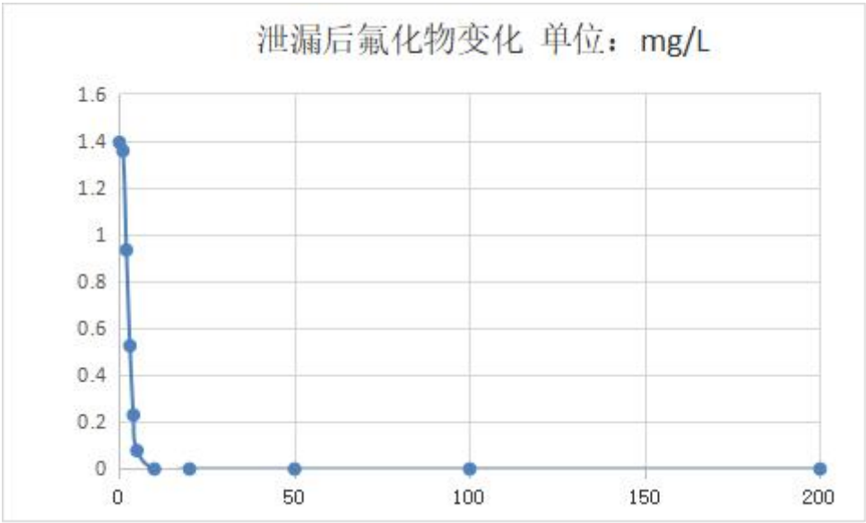
图 5.2-2 非正常状况下氟化物随时间变化曲线图 (单位 mg/L)
