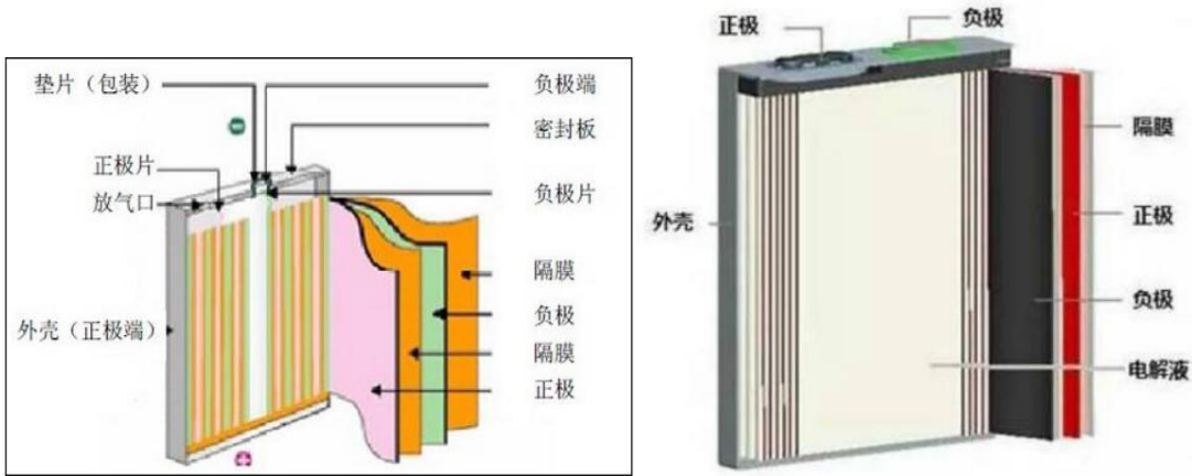
(方形锂电池)
