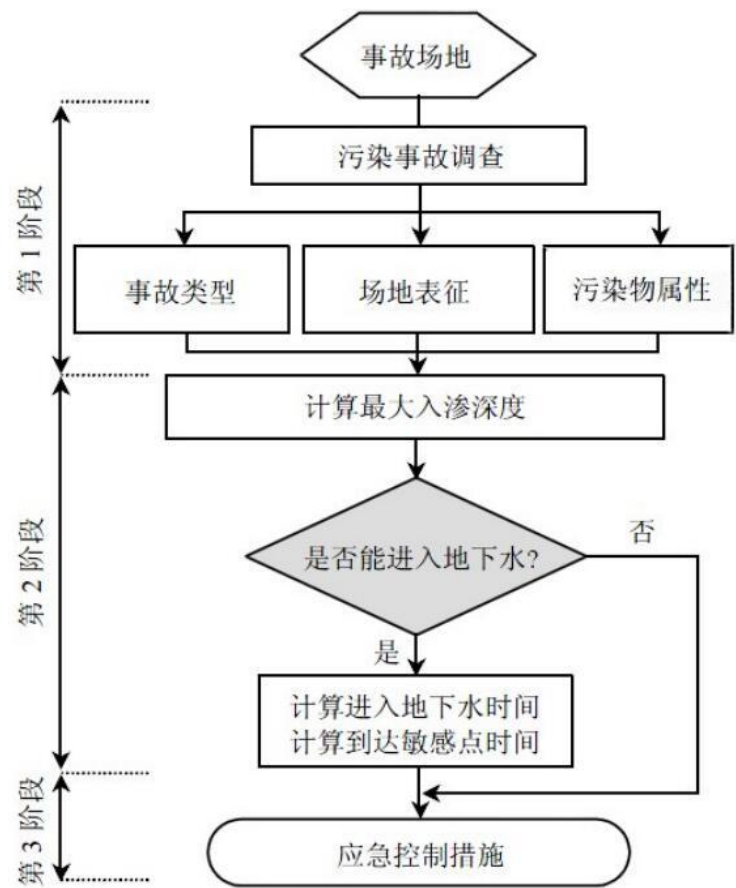
图 6.2-7 地下水污染风险评估流程图
