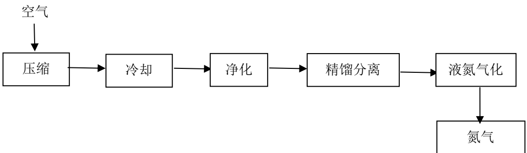
图 3.8-3 制氮站流程
