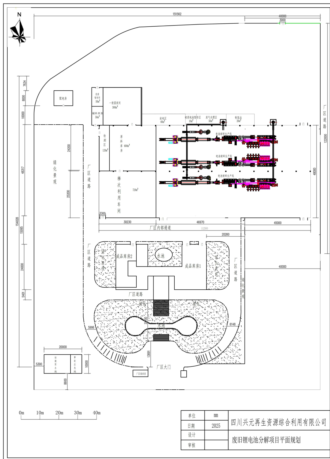
图 3.6-1 厂区平面布置示意图
