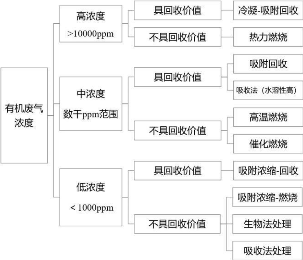
图 6.2-3 VOCs 治理技术适用范围
