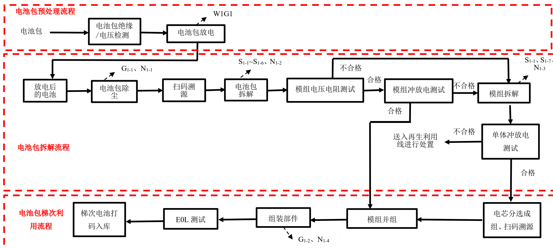
图 3.8-2 废旧锂电池的梯次利用生产工艺流程图及产污节点
