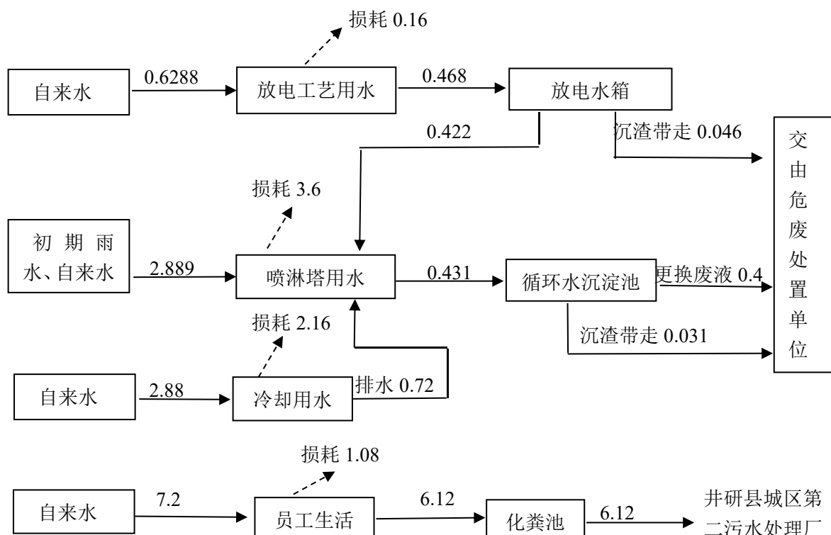
图3.9-3 本项目水平衡示意图 (m³/d)
