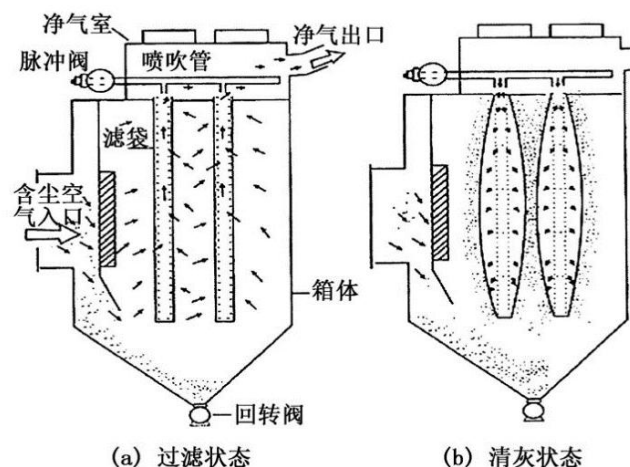
图 6.2-3 布袋除尘器工作原理图
