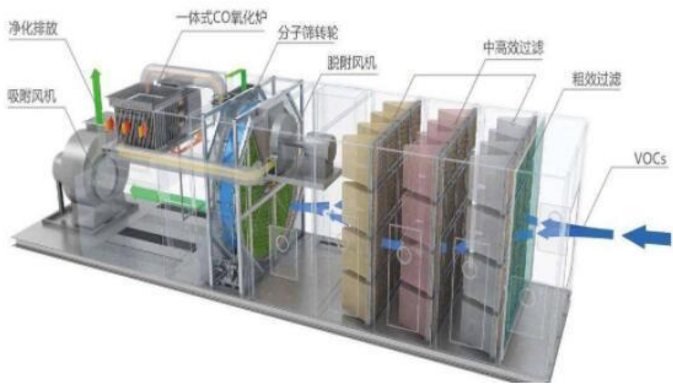
图 6.2-5 沸石转轮吸附+RCO 催化燃烧工艺示意图
