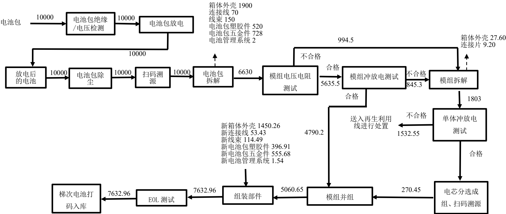
图 3.9-1 废旧锂电池的梯次利用物料平衡图 (t/a)
