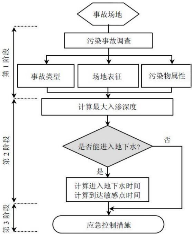
图 5.2-5 地下水污染风险评估流程图
