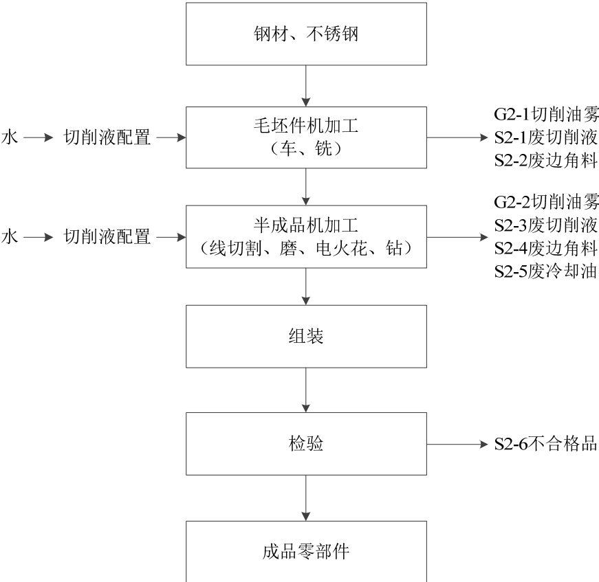
图 2-3 光伏零部件生产工艺流程图
