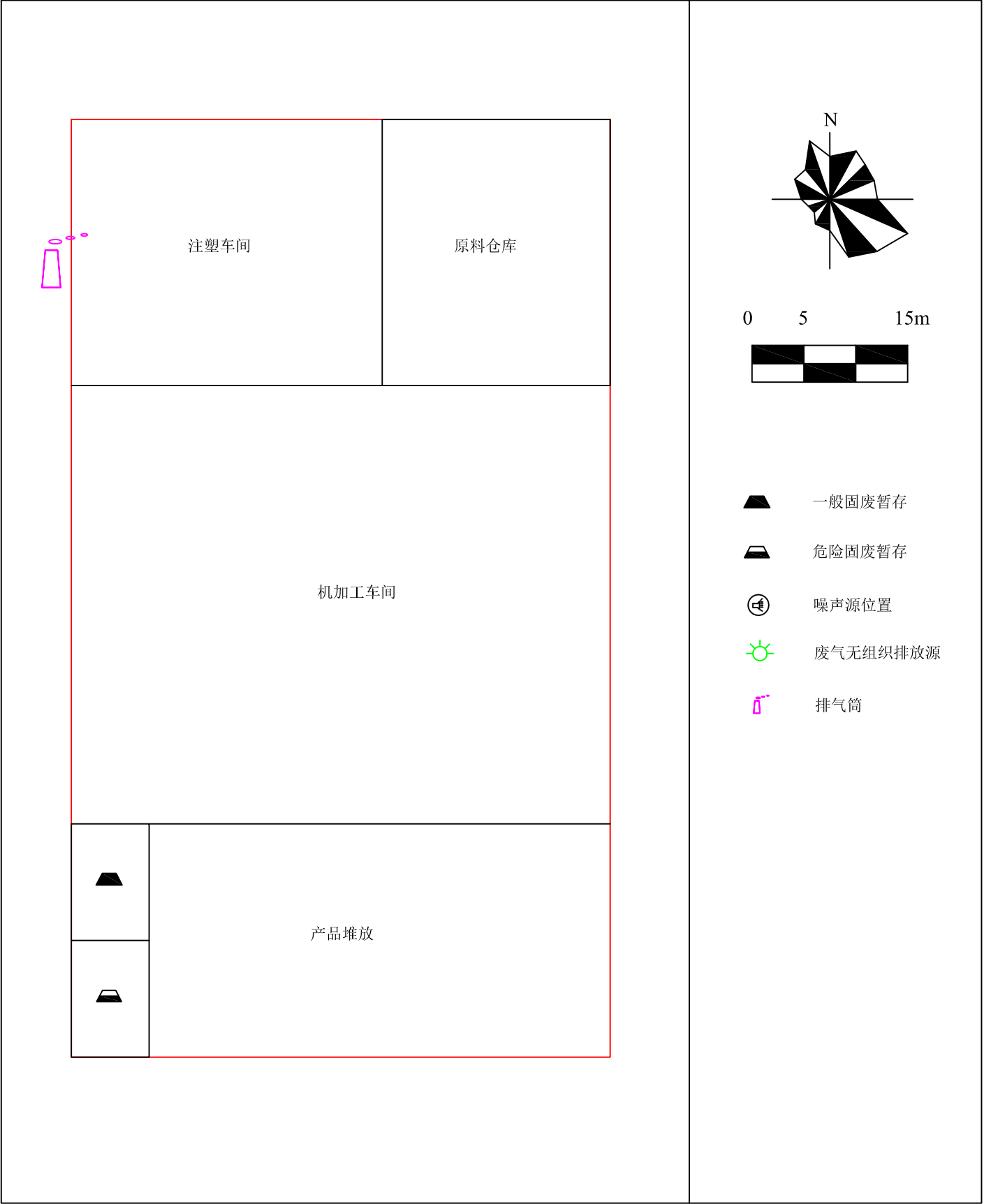
附图8 生产车间平面布置图
