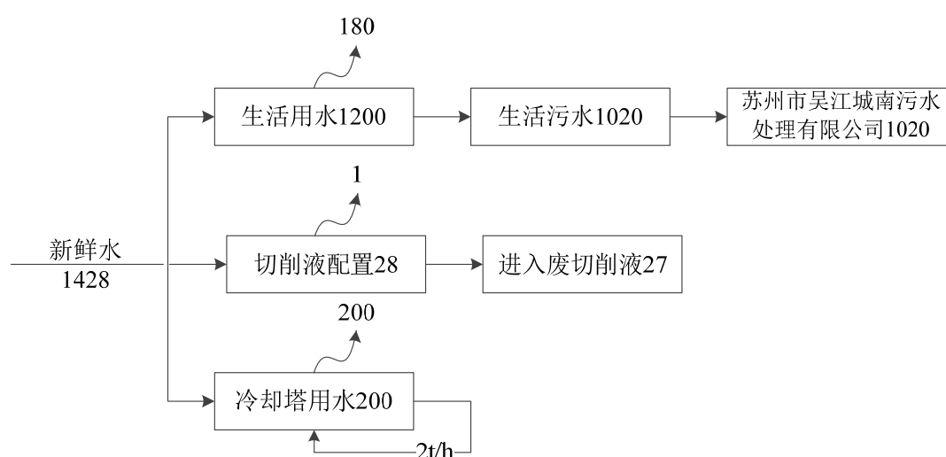
图 2-1 全厂水平衡图 (t/a)
